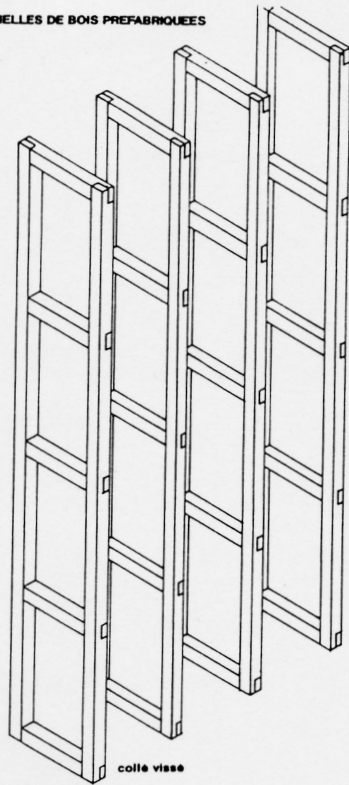
DISPOSITION DES ECHELLES DE BOIS PREFABRIQUEES
