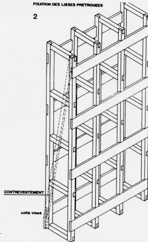
FIXATION DES LISSES PRETROUVEES
